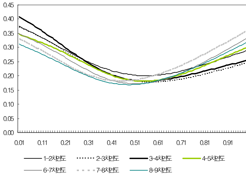
[그림 5-1] 연도별 소득이행변수 분산 곡선의 패턴 변화추이 (단위: \ln^2(\text{만원}) )
