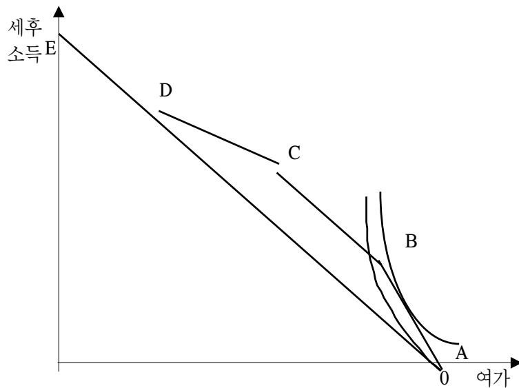
[그림 7-9] 근로장려세제(EITC)에 의한 예산제약식 변화
